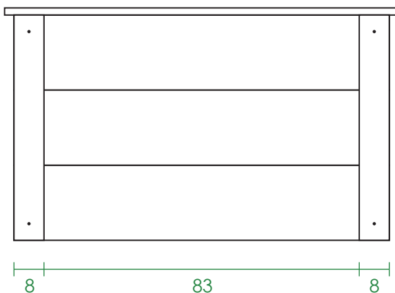
Ansicht Breitseite
